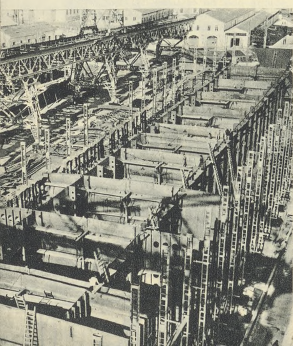
La flota española aumenta su tonelaje. En grada, un nuevo petrolero.
