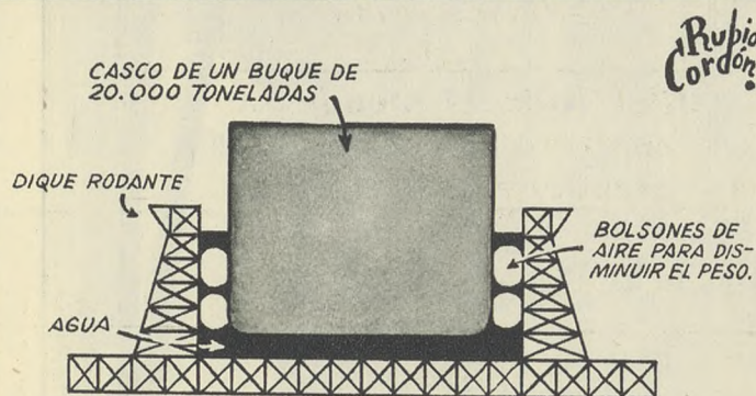
Sección de la caja transportadora, mostrando su estructura y la disposición lateral de las grandes bolsas de aire para disminuir el peso del agua.
