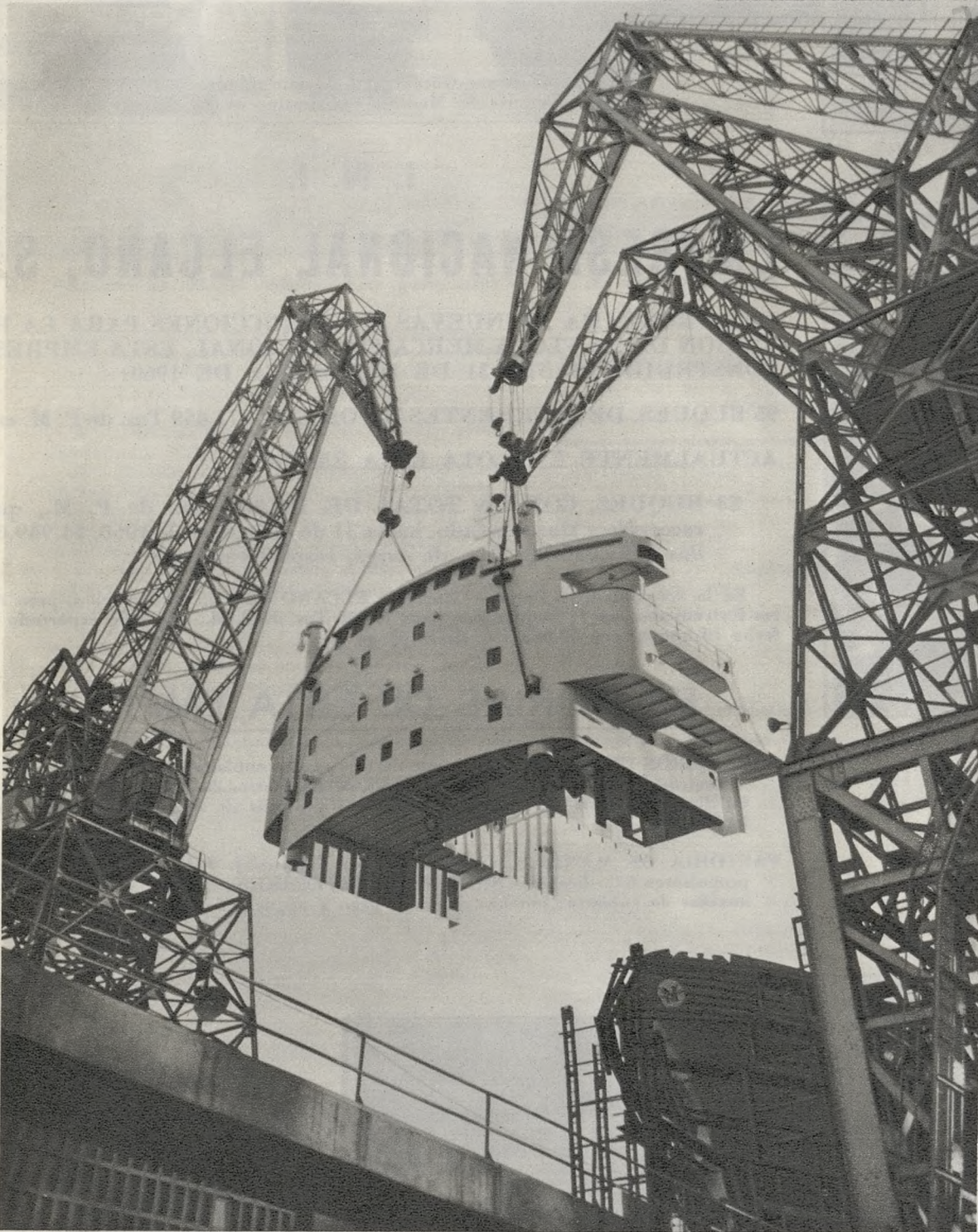
Montaje en grada super-estructura, totalmente terminada, 130 toneladas
