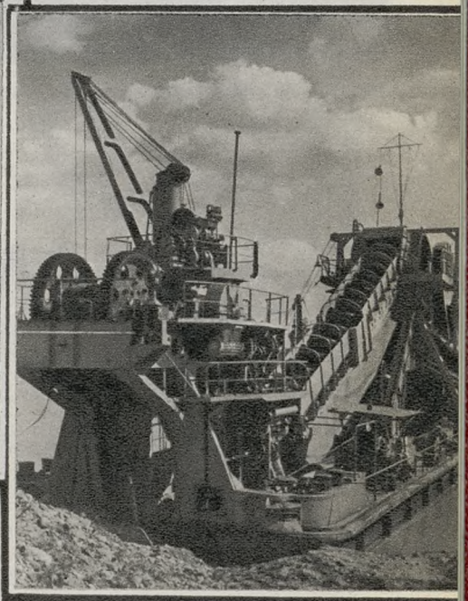
Draga de rosario, de 830 litros de capacidad, de cangilones, construida en Astilleros de Sevilla para la Argentina
