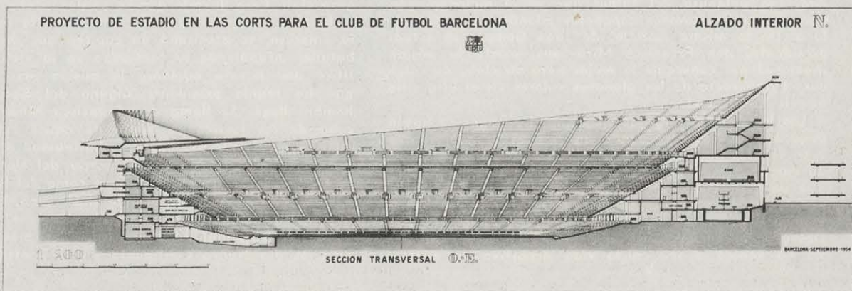
Sección transversal del proyecto para el nuevo estadio, verdadero prodigio de la arquitectura moderna.
