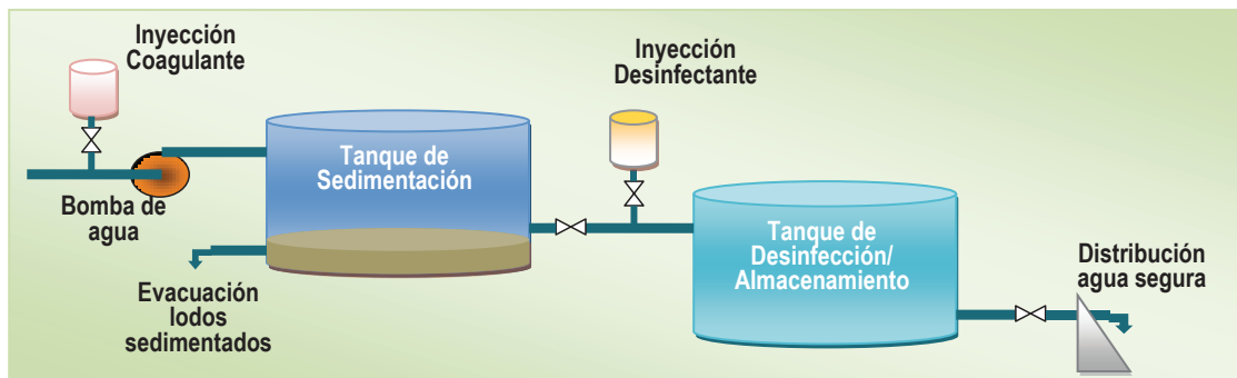
Gráfico 13. SISTEMA BATCH
